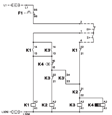
K3Y80 bis K3Y200 Steuerung mit Tastern
