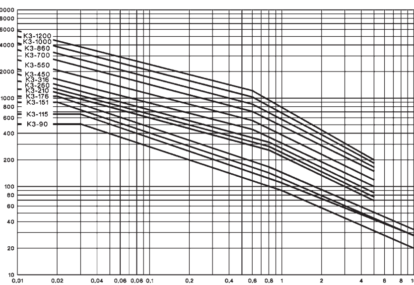
Millionen Schaltspiele
